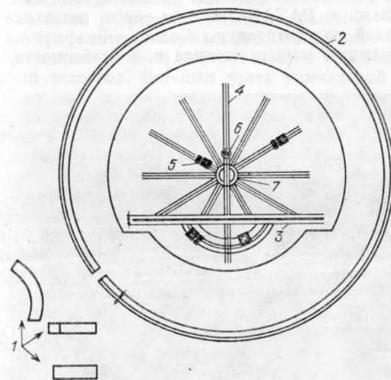
Рис. 39. Схема радиотелескопа РАТАН-600: 1 — лабораторные корпуса; 2 — кольцевой отражатель; 3 — прямолинейный отражатель; 4 — рельсовые пути для перемещения облучателей; 5 — передвижные вагоны-лаборатории с облучателями; 6 — приемник радиоизлучения; 7 — поворотный круг
