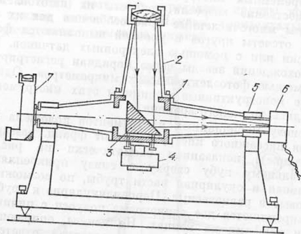
Рис. 23. Схема малого пассажного инструмента: 1 — центральный куб; 2 — верхняя часть трубы с объективом; 3 — диагональная призма; 4 — противовес; 5 — цапфы горизонтальной оси; 6 — блок фотоумножителей; 7 — искатель для наведения инструмента на звезду
