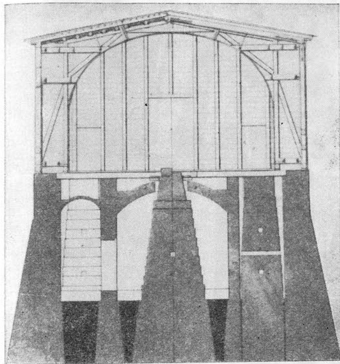
Рис. 11. Фундаменты Пулковской обсерватории. Для придания большей устойчивости астрономические инструменты устанавливаются на массивных каменных столбах, не связанных с фундаментом здания обсерватории
