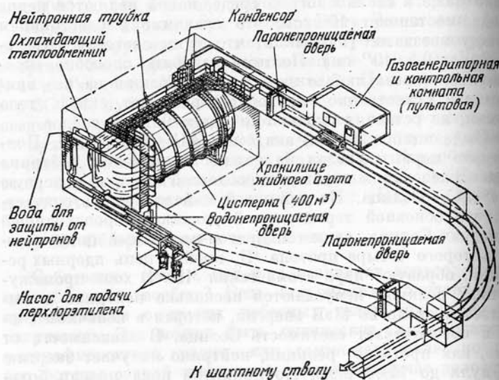
Рис. 82. Схема нейтринного телескопа Дэвиса
