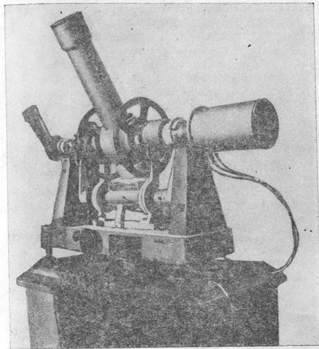
Рис. 24. Малый фотоэлектрический пассажный инструмент АПМ-1
