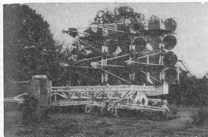
Рис. 81. Высокочувствительный 24-зеркальный гамма-телескоп Крымской астрофизической обсерватории
