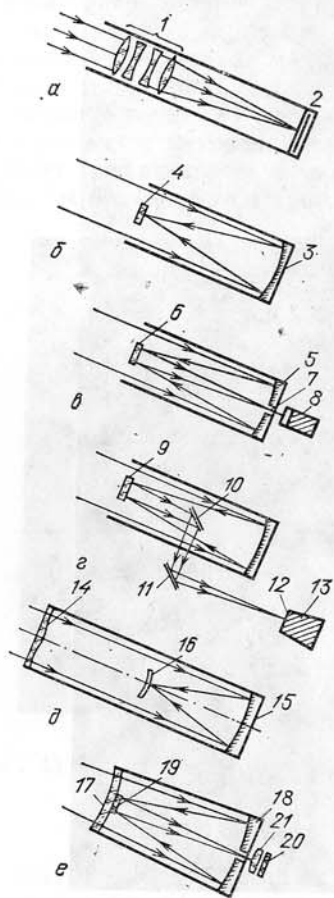
Рис. 15. Оптические схемы телескопов. Обозначения приведены в тексте
