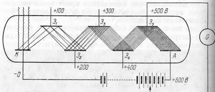
Рис. 19. Схема многокаскадного фотоумножителя: K — фотокатод; \mathcal{E}_1, \dots, \mathcal{E}_5 — последовательно расположенные эмиттеры; A — анод. Количество электронов, попадающих на анод, в 10^6 – 10^9 раз больше числа электронов, выделенных катодом ФЭУ
