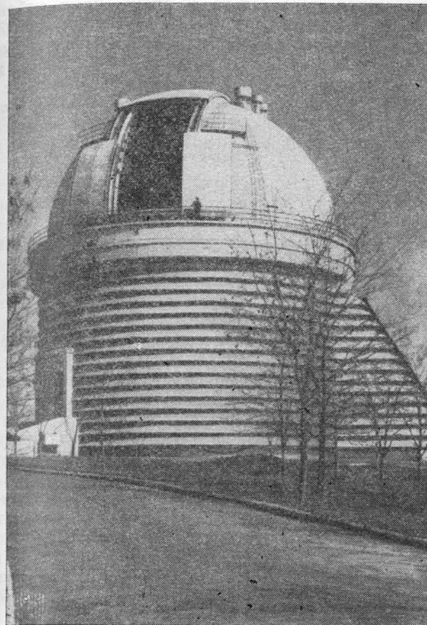
Рис. 56. Башня ЗТШ. Выступ справа соответствует оптическому каналу схемы кудэ
